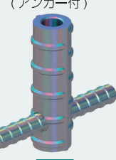
《Oインサート》
