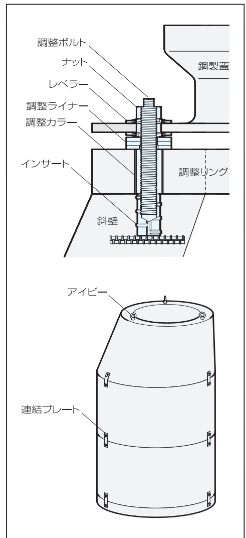
《SUSインサート》
